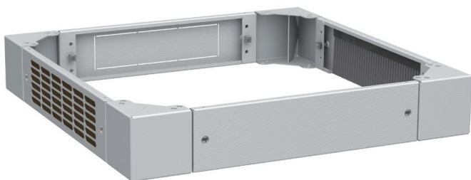
Příklad sestavení podstavce výška 100 mm, šířka 600 mm, hloubka 600 mm
